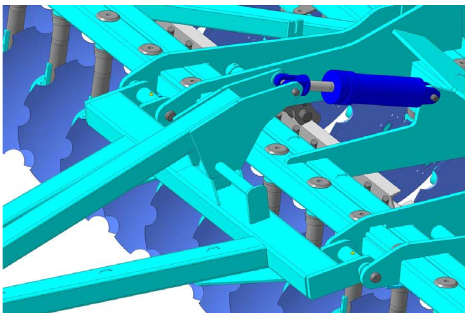
Усиленная треугольная сница
