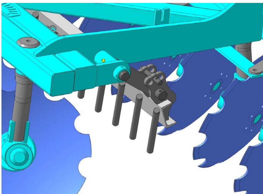
Усиленная треугольная скоба
