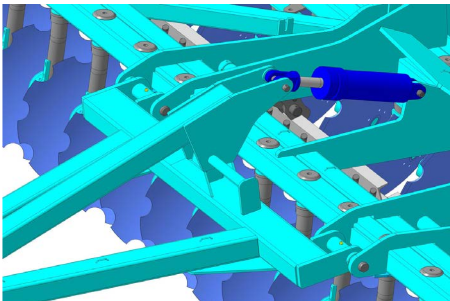
Усиленная треугольная скоба
