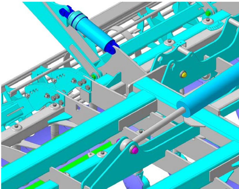
Модернизированная ходовая тележка
